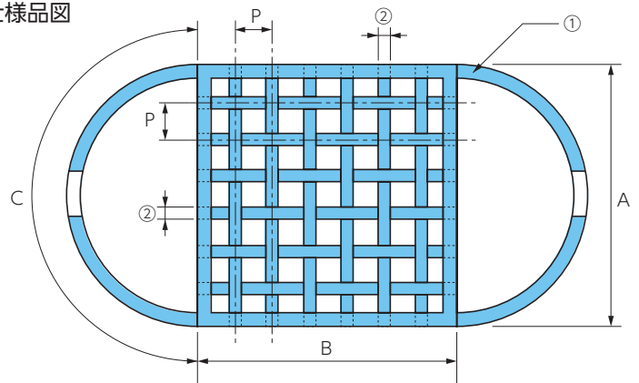
標準仕様品図
